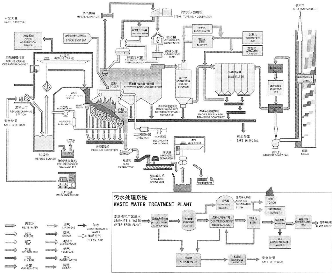
工艺流程图
